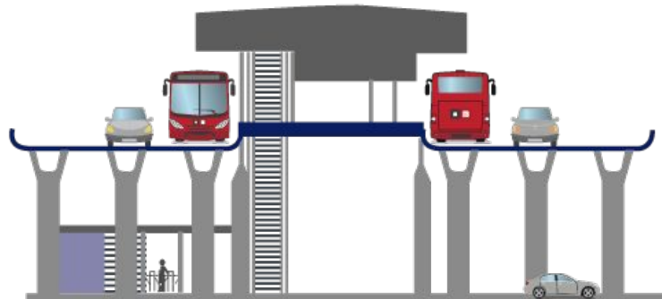
Estaciones elevadas en puentes vehiculares (doble acople)
