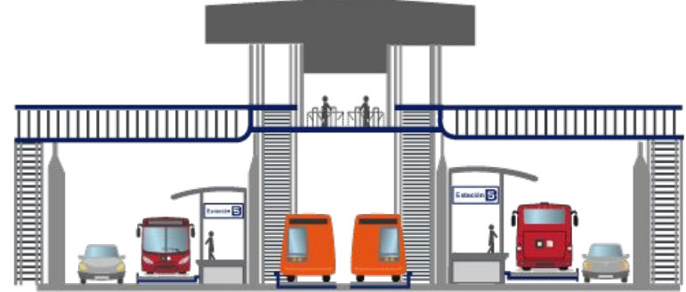
Estación con un acople de autobús por sentido de vialidad
